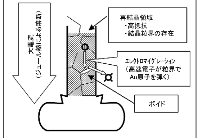
図9. 樹脂の熱膨張によりAuワイヤーにかかる応力
